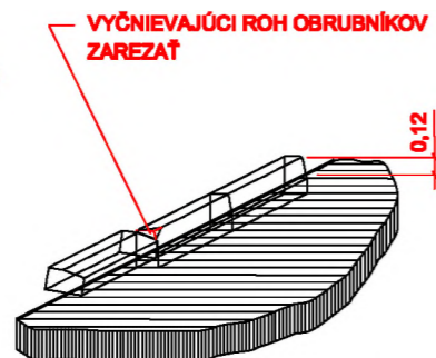
DETAIL - OBRUBNÍK NA STOJATO / NA LEŽATO
